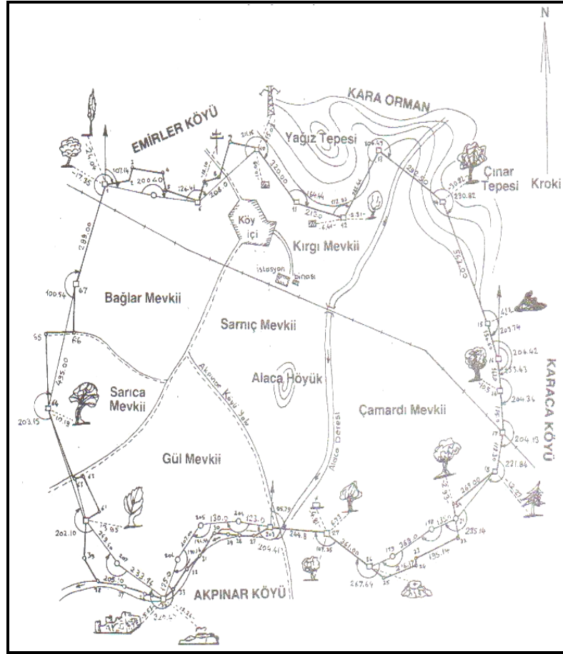
Kroki 1.2: Köyler için düzenlenen kadastro alanı kroki
