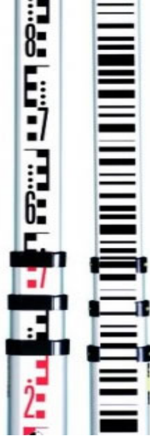
Fotoğraf 2.23: Mira ve barkotlu mira
